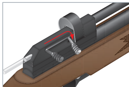
9. Faites passer le levier verrou [levier d'armement] en avant et vers le bas pour le fermer. N'introduisez jamais plus d'un diabolo dans le canon. Pour empêcher le chargement de deux diabolos, il est conseillé de n'introduire le diabolo dans le canon que juste avant le tir.
